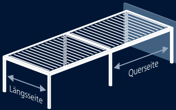
Kopplung in Querrichtung (Anlagen voreinander an der Wand) max. 24 Meter
