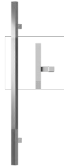
Pageno Edelstahl poliert und matt, Länge: 1000 mm, gerade Stützen für Griffmontage auf flügelüberdeckender Türfüllung, optional mit abgewinkelten Stützen für Montage auf Türflügel
