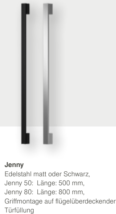
Votan Edelstahl matt oder Schwarz, Längen: 800, 1000, 1200, 1400, 1600 und 1800 mm, Griffmontage auf flügelüberde- ckender Türfüllung
